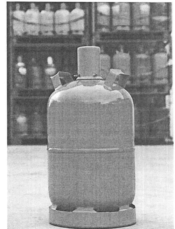
Flüssiggasflasche mit Schutzkappe für Transport und Lagerung
